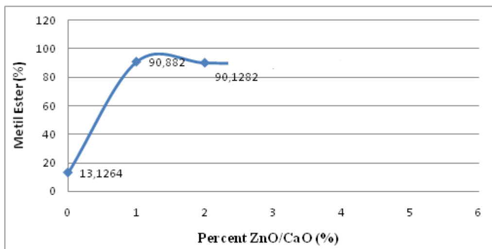
Fig-3: Percent ZnO/CaO (%) vs Metil Ester (%)
